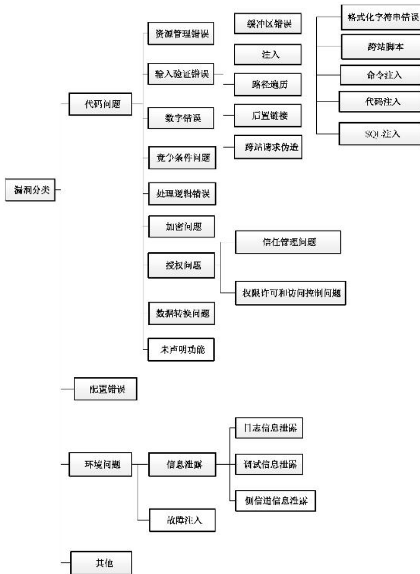
图 1 网络安全漏洞分类导图
