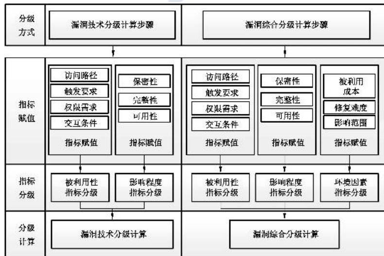
图 2 漏洞分级过程示意图
