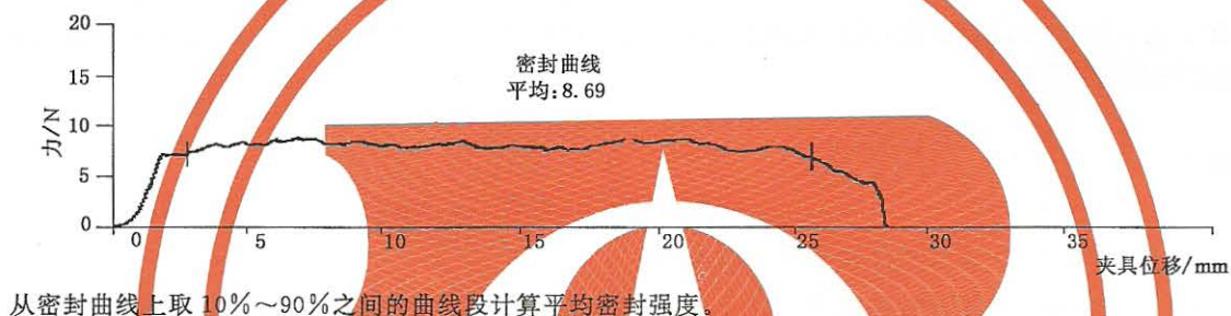
图3 平均密封强度的计算
