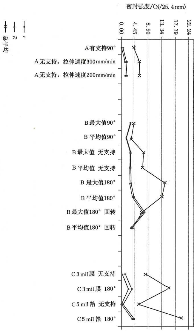
图 C.1 实验室协同研究的 r 和 R (在 95% 的置信度) 和测得均值
